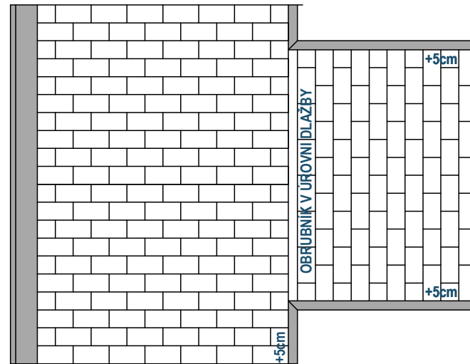
"T" NAPOJENÍ DLAŽBA - VJEZD, VSTUP K RD A POD.
